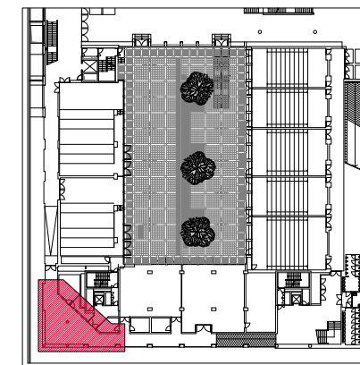
U1 - PIANTA PIANO PRIMO INTERRATO
