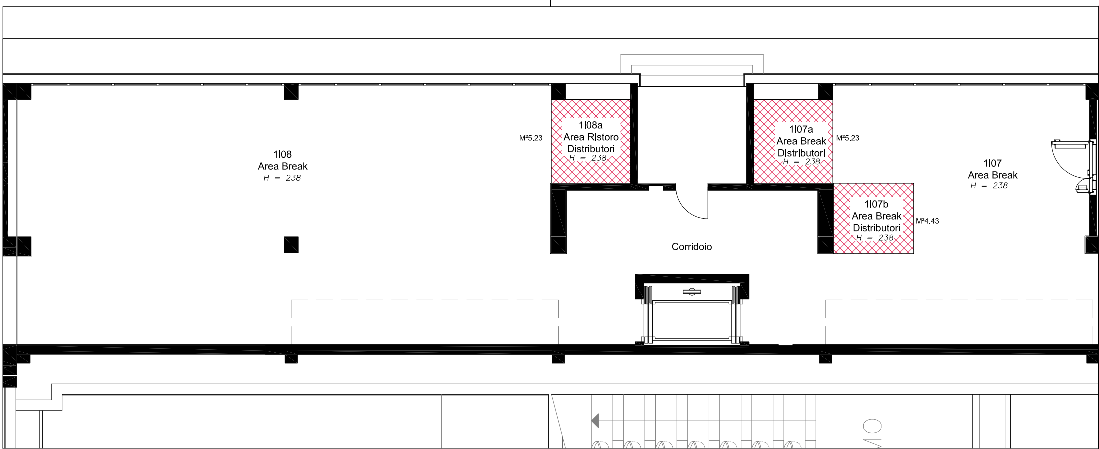
U9 KOINE' - Pianta Piano Primo Interrato - Locale 1i07b, 1i07a e 1i08a
